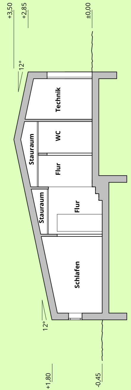
Längsschnitt
