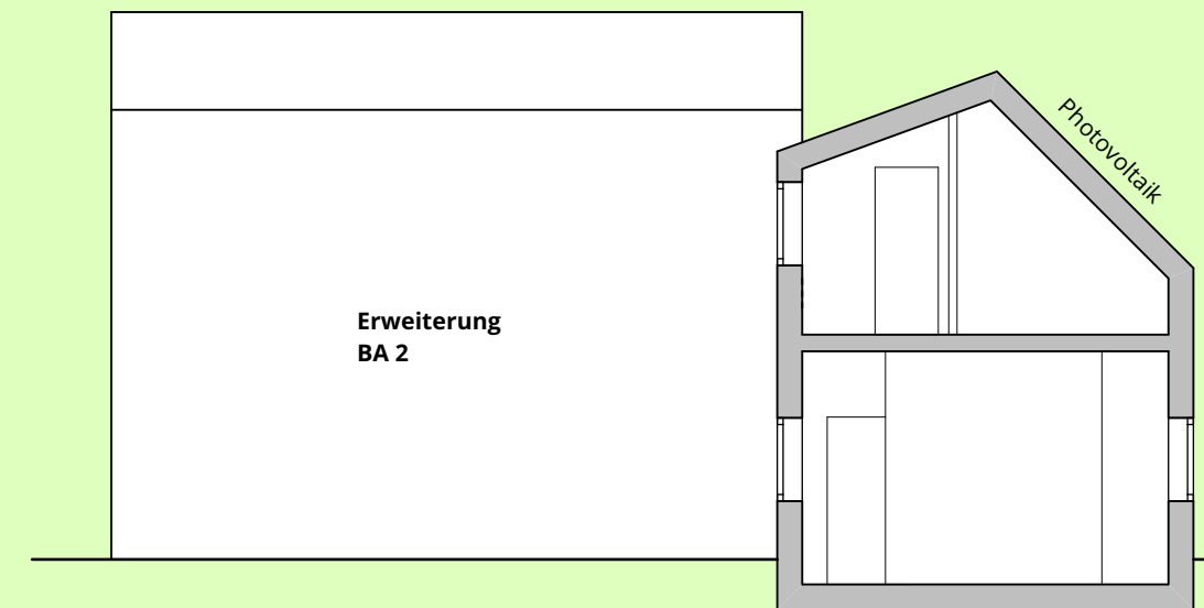
Schnitt Starterhaus (BA1)
