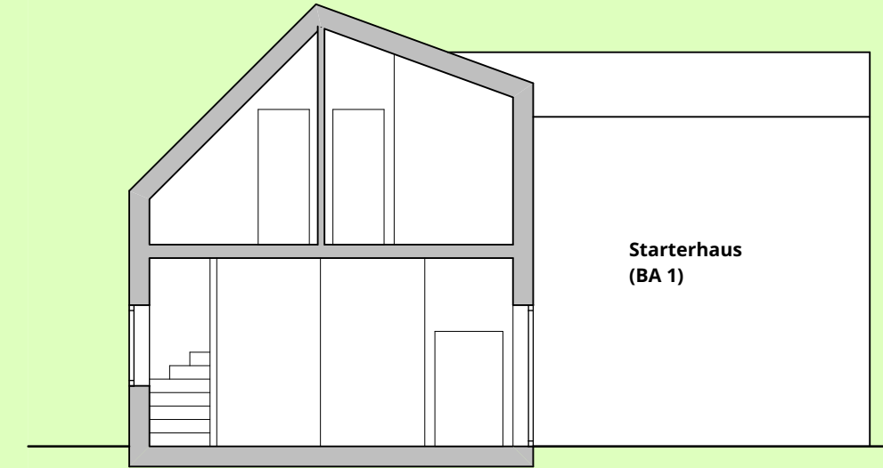
Schnitt Erweiterung (BA2)
