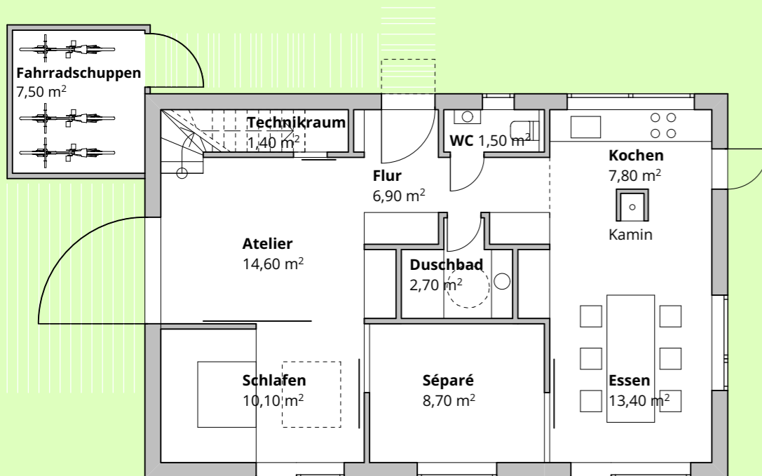
Erdgeschoss
