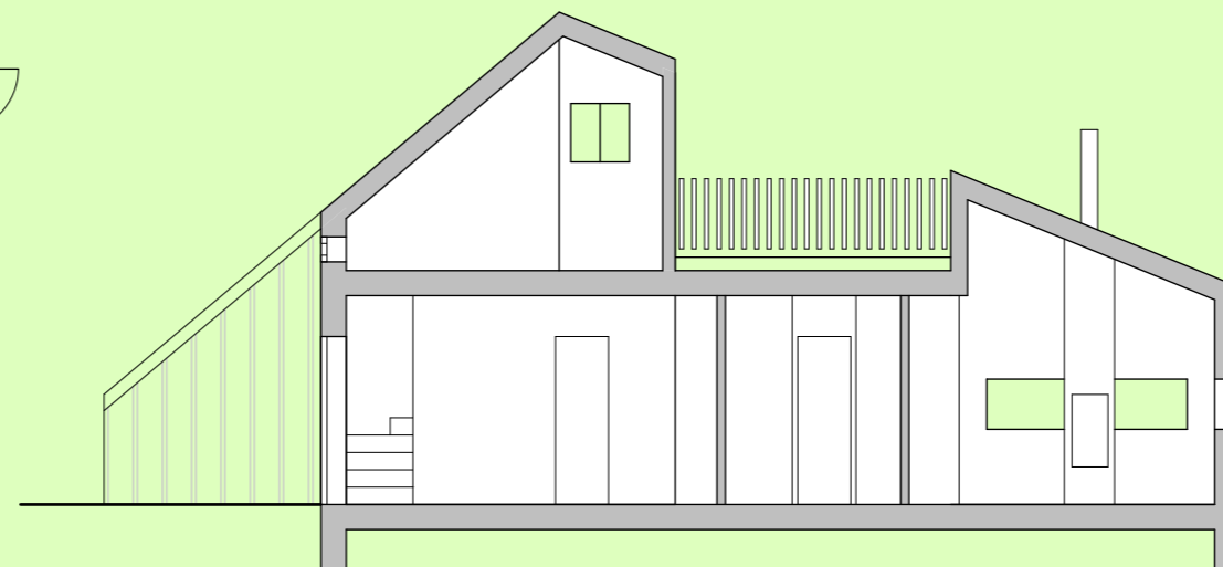
Querschnitt
